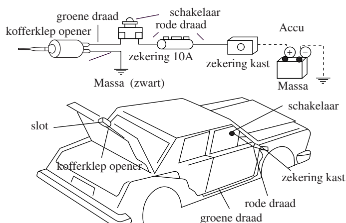
Fig. D Installatie diagram
